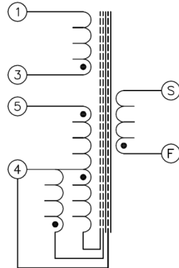
Электрическая схема
