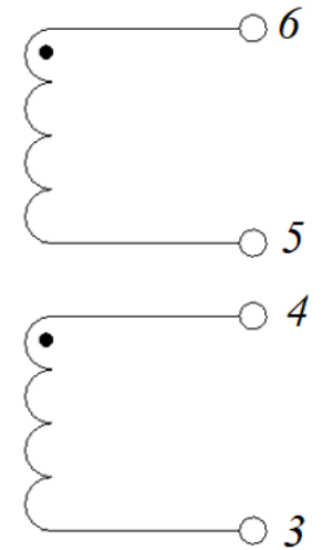
Электрическая схема
